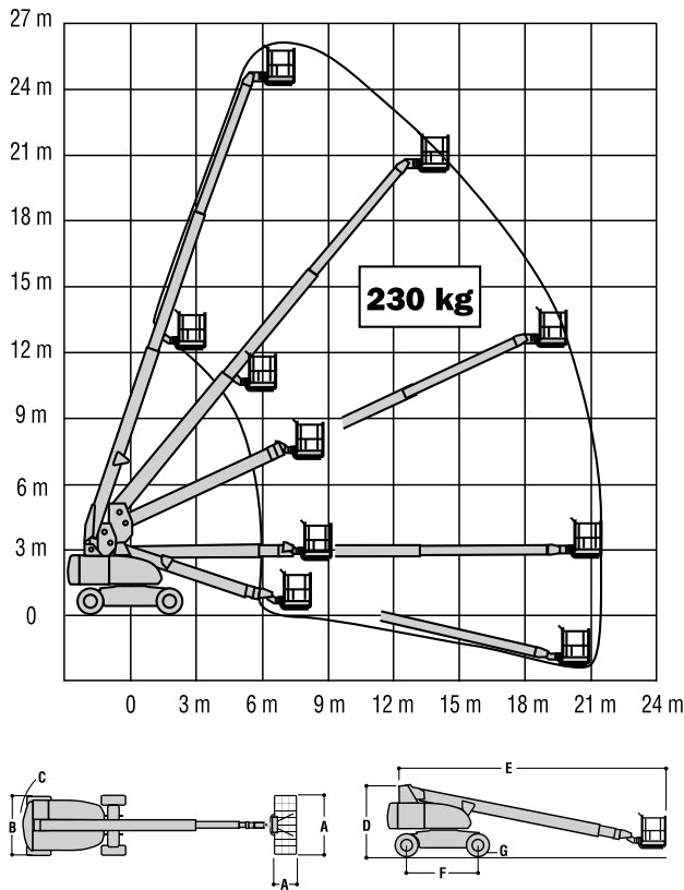
800S JLG modell
